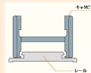
レール断面
